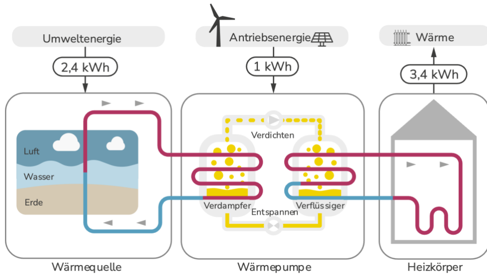
Abbildung 7: Gesamteffizienz einer Wärmepumpe mit Arbeitszahl = 3,4 (unsaniierter Altbau)
