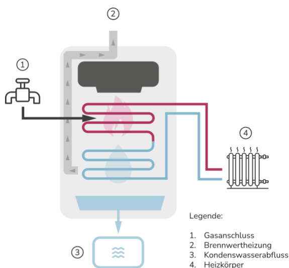
Abbildung 6: Funktionsweise Brennwerttherme
